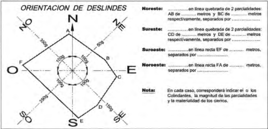
Figura 16. Orientación de los deslindes con vientos intermedios.
