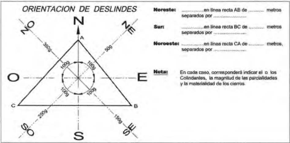
Figura 17. Orientación de los deslindes para predio triangular.
